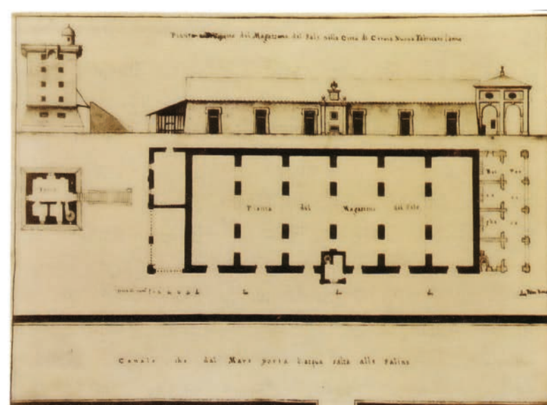
Cervia (RA), »Magazzino Torre« (»Skladišče Stolp«), tloris in pročelje skladišča (iz Storia di Cervia (»Zgodovina mesta Cervia«), druga knjiga, Rimini 1998, Album imperiali, privatna zbirka)
